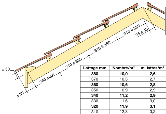
COTATIONS SUR RAMPANT - Pureau variable (tolérance lattage ± 2 mm)
